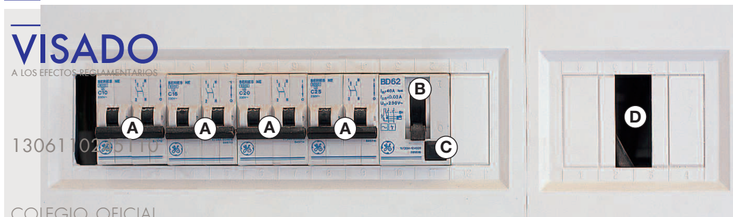
11. CUADRO DE PROTECCIÓN INDIVIDUAL: A. Pequeños interruptores automáticos (PIA). B. Interruptor automático diferencial (IAD). C. Botón de prueba. D. Alojamiento del interruptor de control de potencia (ICP).
